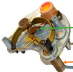
Innenleben der Benzin- und Öldruckanzeige
