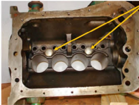
Topolino- Motorblock von unten bei ausgebautem Innenleben
