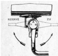
Abb. 11 A. Kraftstoffbehälterhahn (auf). A = auf; C = zu; R = Reserve.
