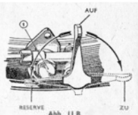
Abb. 11 B. Kraftstoffhahn, in Offen-Stellung. (für Wägen ab Nr. 071000). 1. Haltebefestigungsbohrung. Nach Abschrauben dieses kann der Hahn abgenommen werden.
