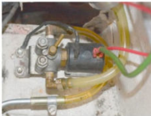
Sperrventil in der Benzinleitung
