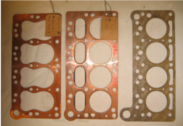
Drei Zylinderkopf-Dichtungen im Vergleich: Topi A (l), Siata (m) und Topi B/C (r)
